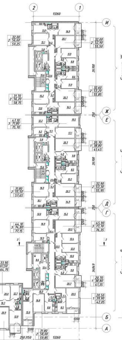
Схема плана типового этажа
